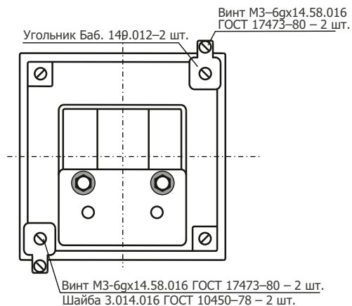
Схема 2. Способ крепления приборов ЭА120Ц, ЭВ120Ц.
