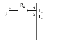
Подключение вольтметра постоянного тока, работающего с добавочным сопротивлением R_d
